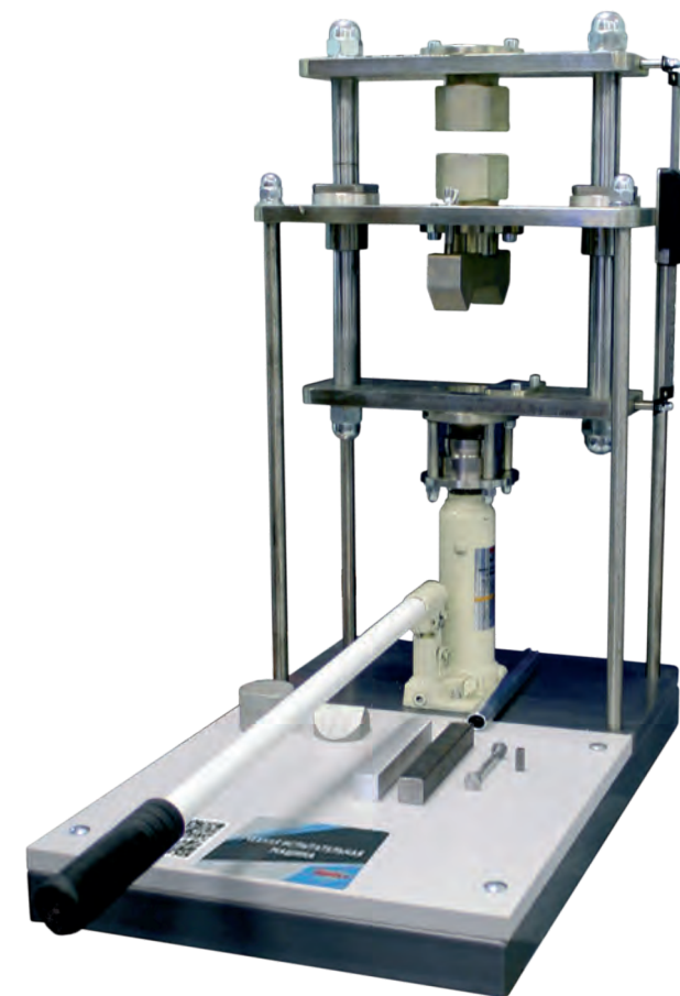
УП6415 Комплект учебно-лабораторного оборудования «Механические свойства материалов» (компьютерная версия)
