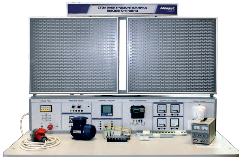
УП5042 Комплект учебно-лабораторного оборудования «Стол электромонтажника высшего уровня» (СЭМВУ-НР-3)
