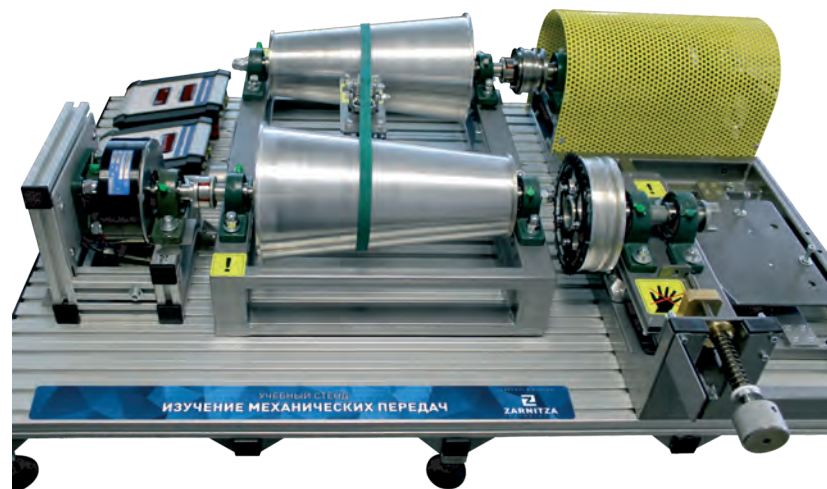
УП5919 Комплект учебно-лабораторного оборудования «Детали машин. Изучение механических передач»
