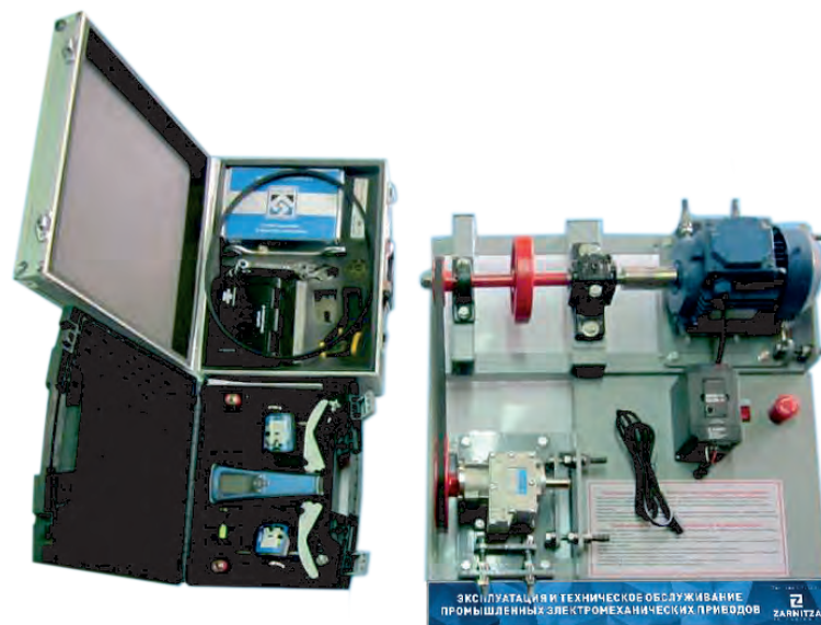
УП5116 Комплект учебно-лабораторного оборудования «Эксплуатация и техническое обслуживание промышленных электромеханических приводов» (ЭиТОПЭП)
