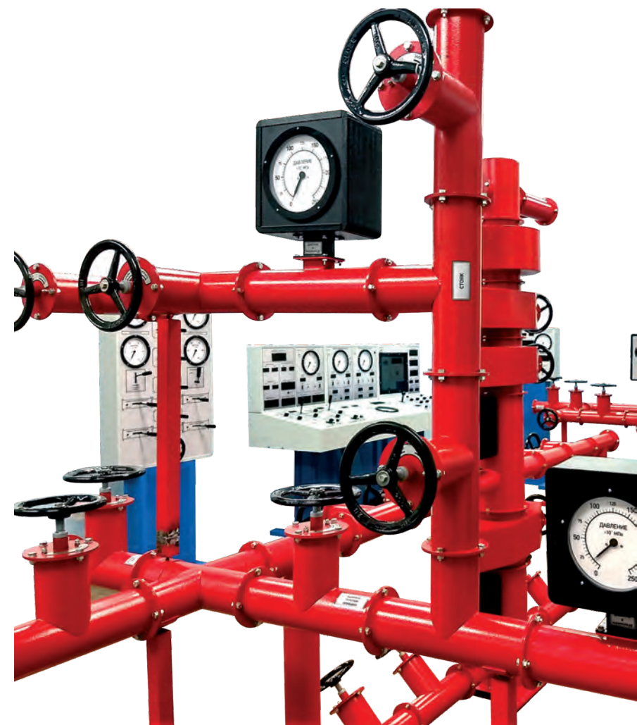
НГ0221 Мобильный буровой тренажер
