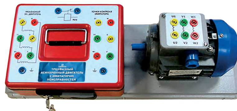
УП5045 Комплект учебно-лабораторного оборудования «Трехфазный асинхронный двигатель с имитатором неисправностей» (ТАДИН)
